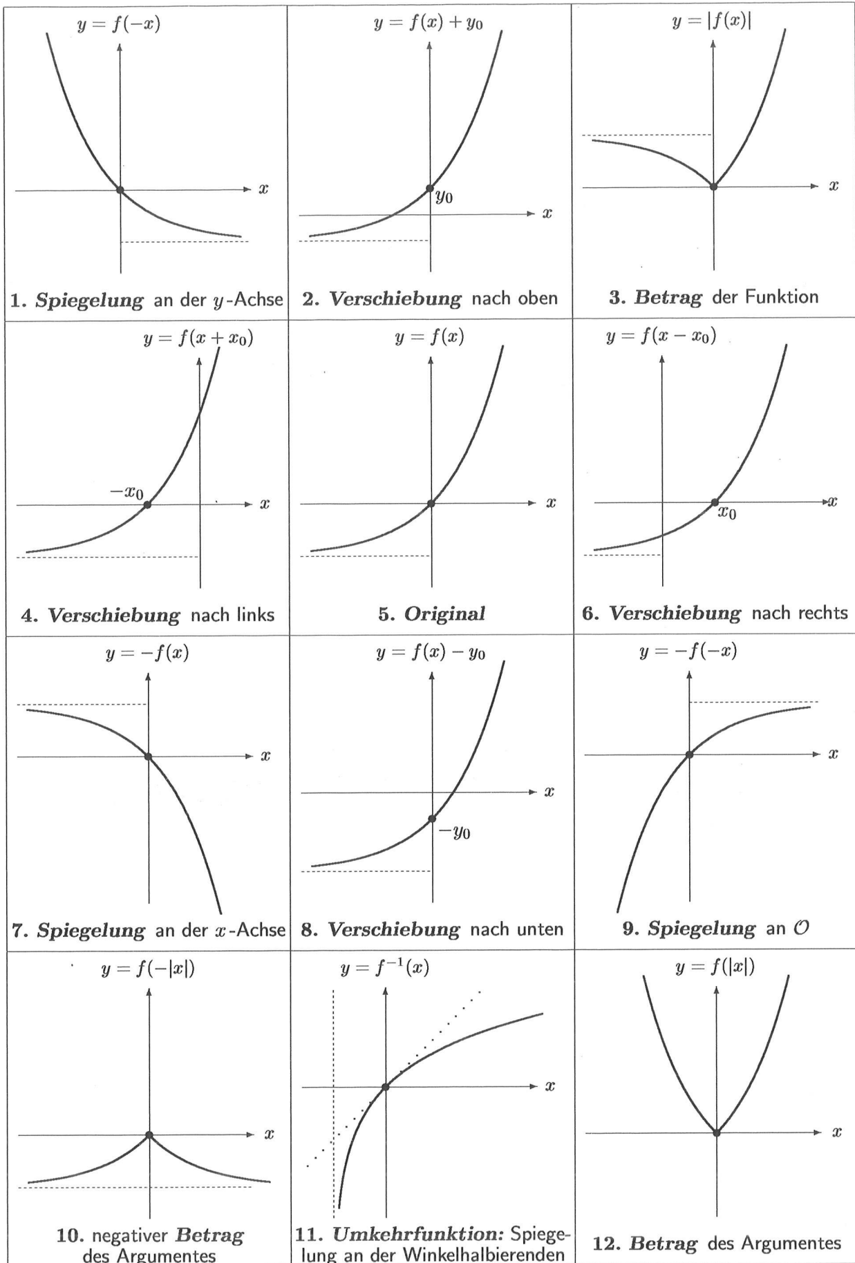
Abbildung 2.12 Verschiebungen und Spiegelungen.
