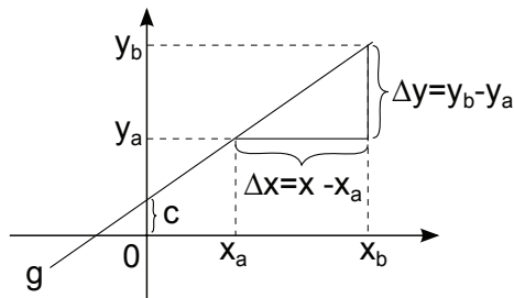
Abbildung 14.1: Geradensteigung und Differenzenquotient
