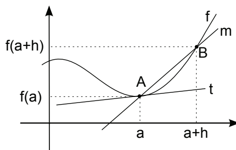
Abbildung 14.3: Die mittlere Änderungsrate m der Funktion f wird zur Tangente t für h \rightarrow 0
