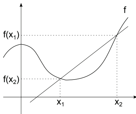
Abbildung 14.2: Mittlere Änderungsrate der Funktion f
